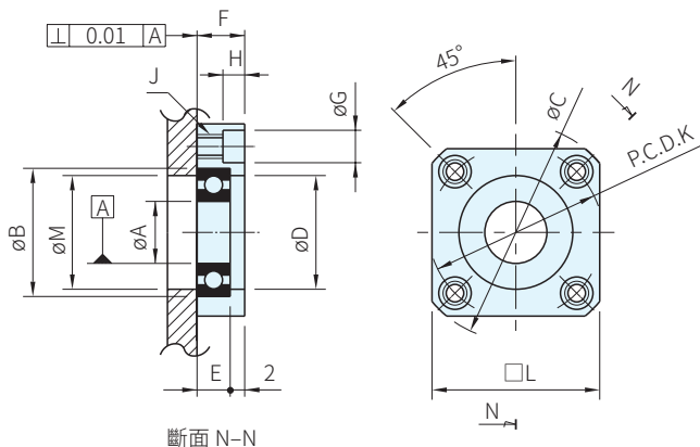
斷面 N-N
